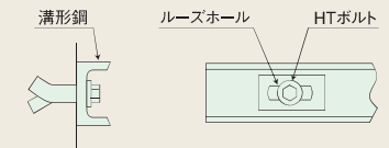
詳細図
