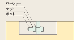
ボルト接合部詳細図
