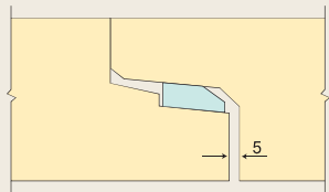
継手部詳細図
