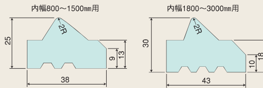
継手用ゴム輪
